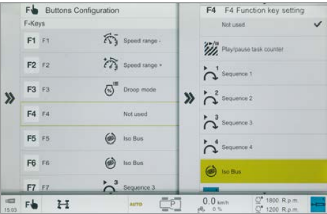
F-toetsen toekenning in de CEBIS
