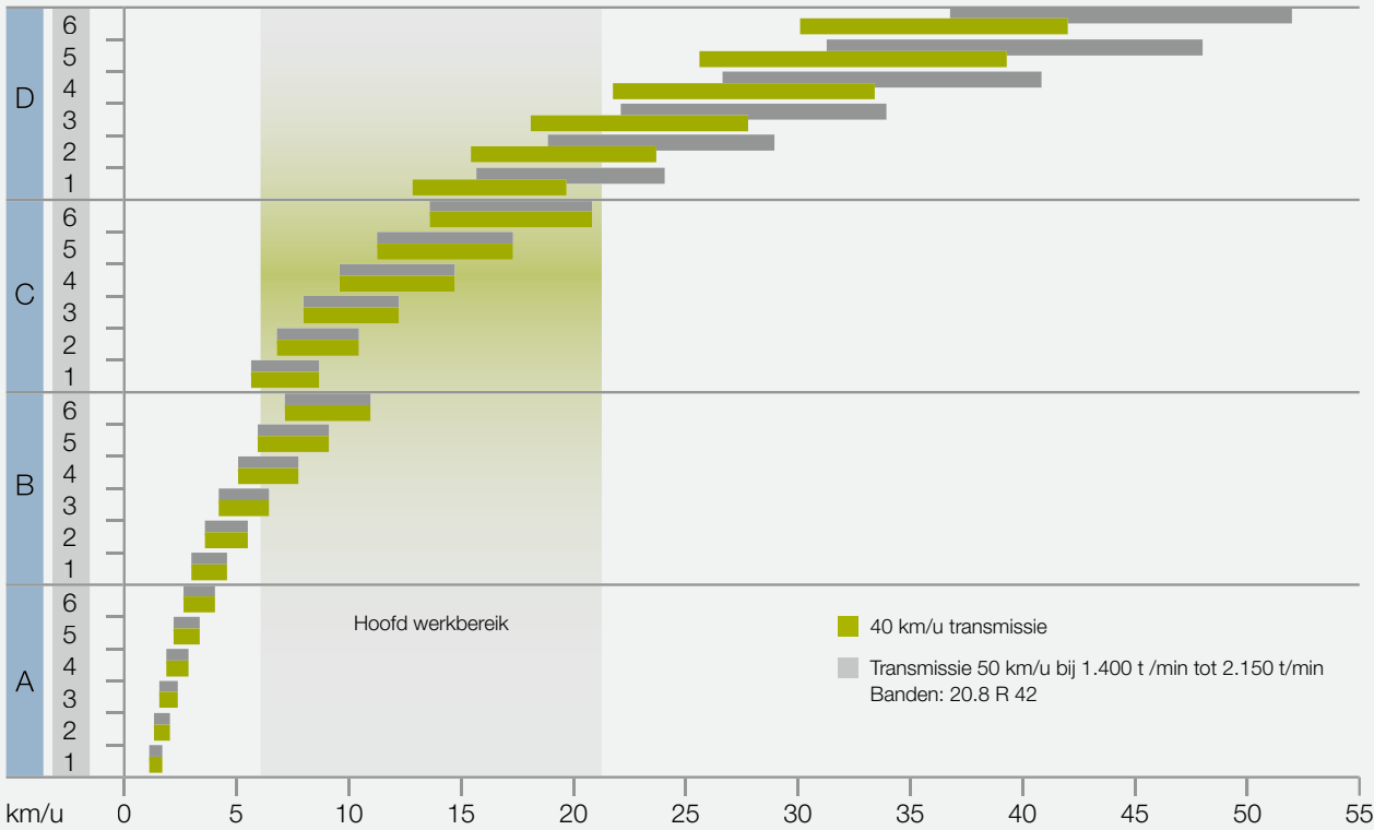
HEXASHIFT: 24 versnellingen voor optimale snelheidsverdeling
